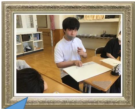
ブラックホール
